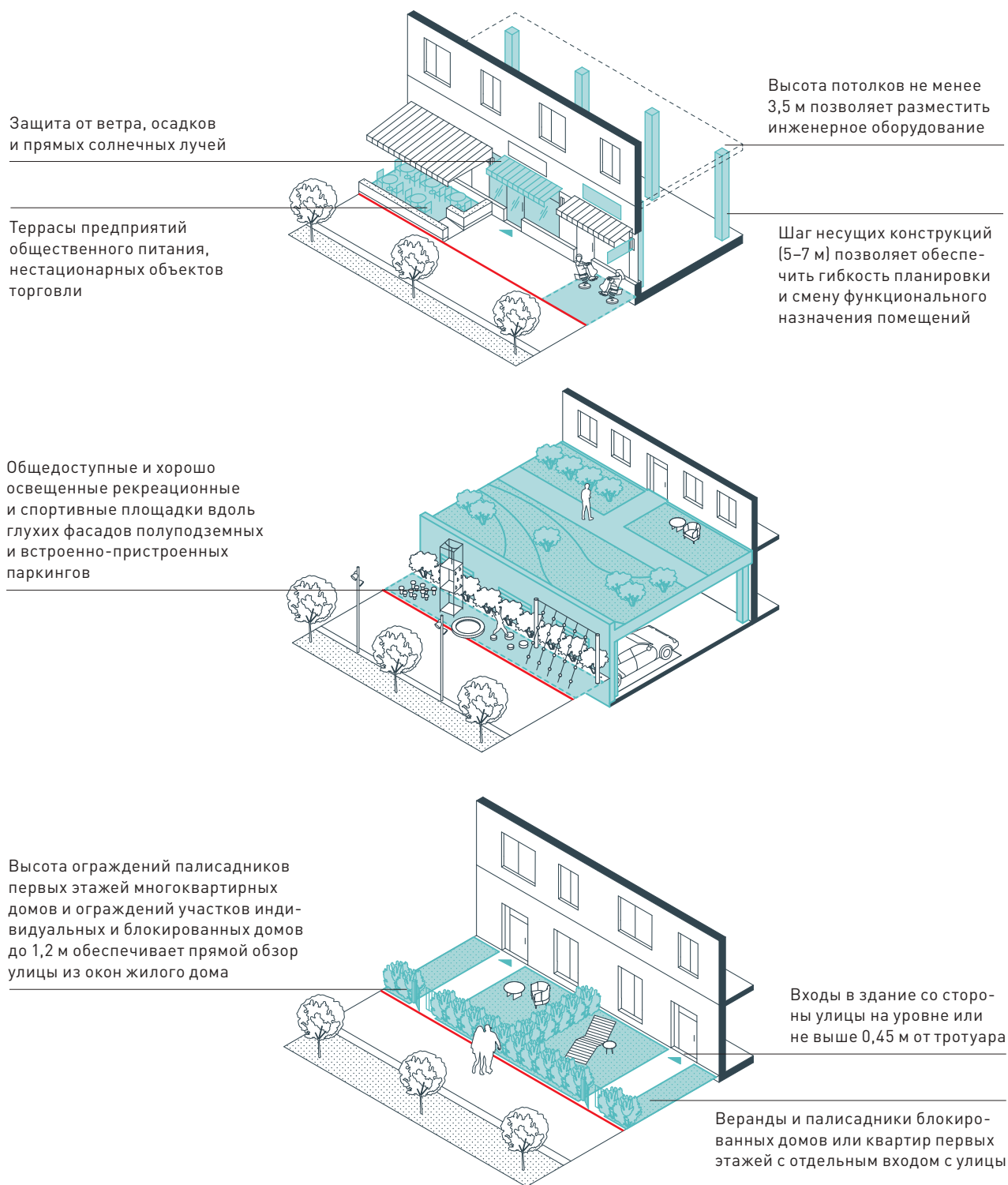
Илл. 22. Устройство уличного фронта и прифасадной зоны
