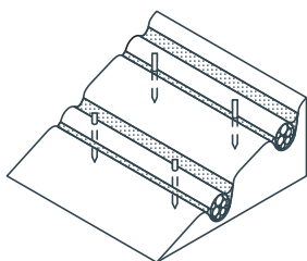
3 Фаширование (легкие/тяжелые фашины)
