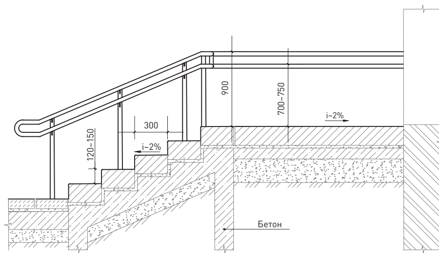
Сечение 2-2
