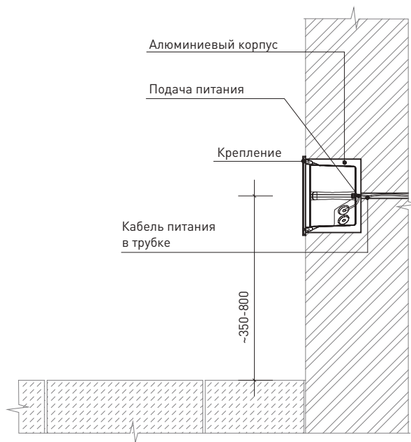
98 Схема установки встроенного светильника на стену / сечение
