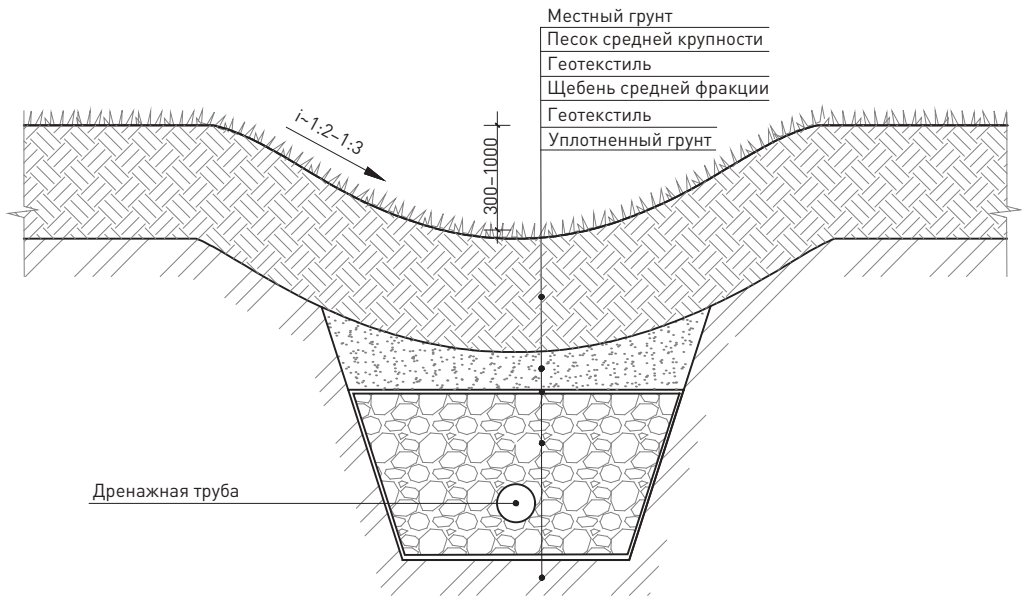
114 Схема устройства биодренажной канавы / сечение
