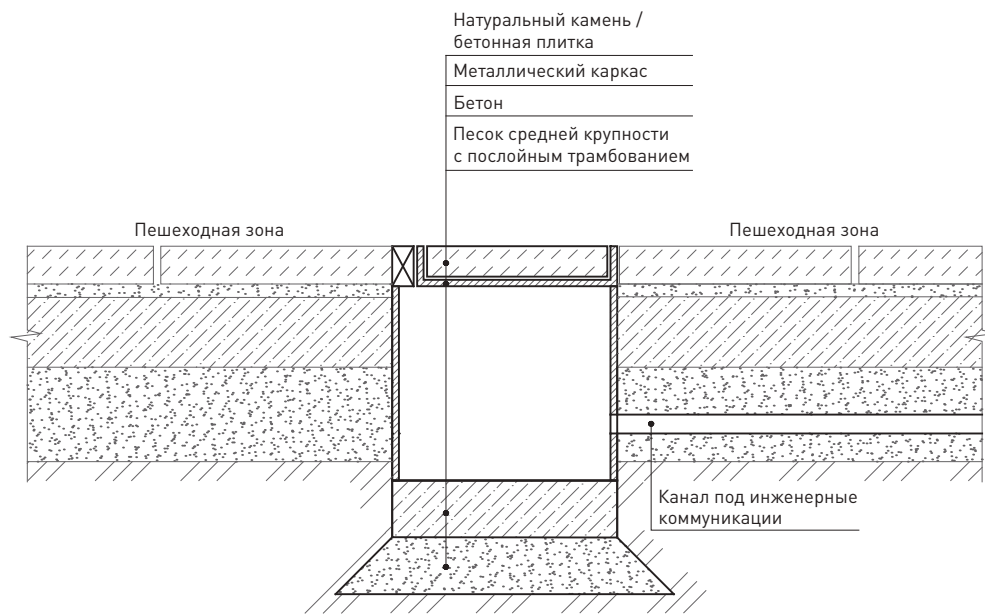
113 Схема устройства приемки подключения к подземным коммуникациям / сечение
