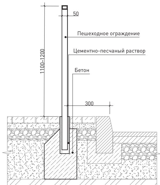
49 Схема установки пешеходного ограждения на тротуаре
