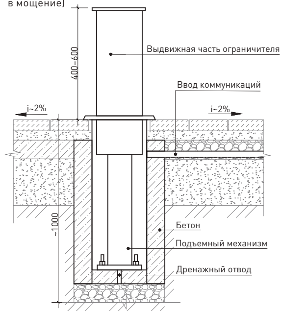
55 Схема установки электромеханического болара (выдвижного ограничителя в мощность)
