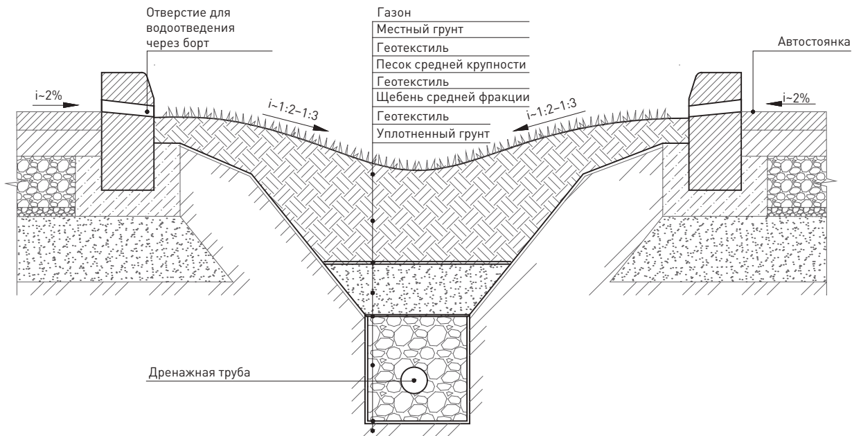
116 Схема устройства биодренажной канавы, отводящей воду от автостоянки / сечение
