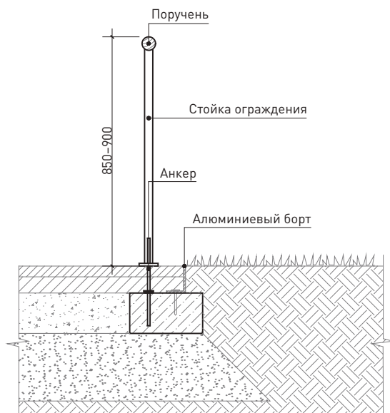
51 Схема установки пешеходного ограждения на эскапаторе
