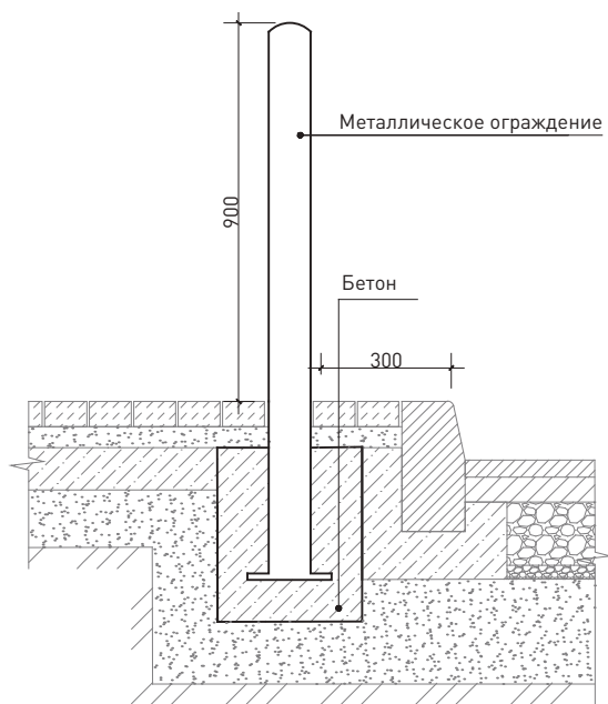
52 Схема установки стального ограничителя парковки
