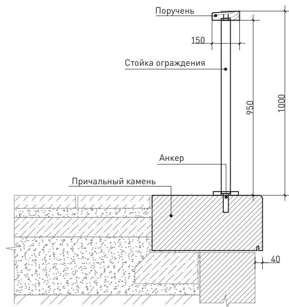
61 Схема установки пешеходного ограждения набережной
